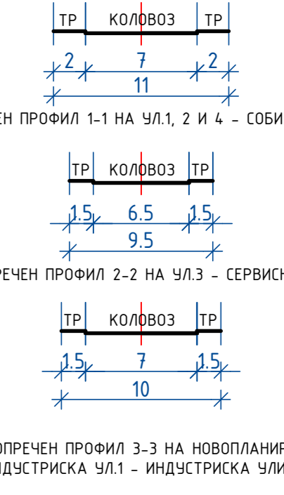
ПОПРЕЧНИ ПРОФИЛИ НА СООБРАЌАЈНИЦИ
